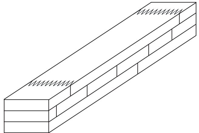
Möglicher Aufbau einer NO LIMITS Kantele
